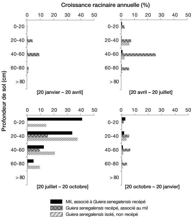
Figure 12.2. Dynamique racinaire moyenne (2013-2015), exprimée en % de croissance racinaire annuelle sur tout le profil, de touffes de G. senegalensis recépées, du mil poussant à proximité et de touffes isolées et non-recépées (n=3, Keur Matar).
